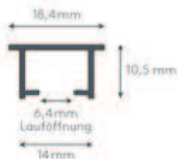
Querschnitt HM110
