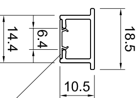
Kunststoffkeder für Lauföffnung
