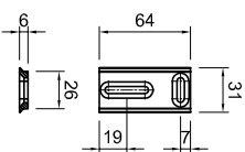
Montageplatte für Wandträger
