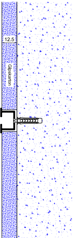
Montage zwischen Gipskartonplatten
