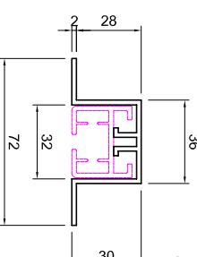
Seitenansicht quer Einbauprofil
