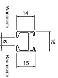
Detail Schiene Modell TOP 455
